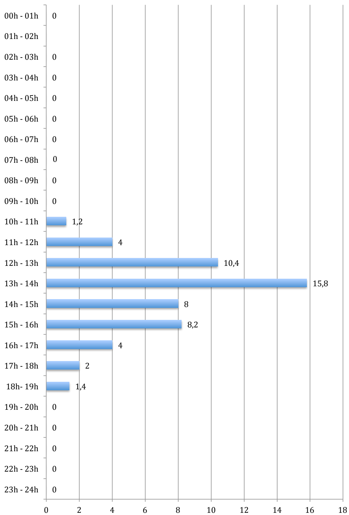
Cantidades de lluvia registradas por horas en CATADAU el día 18/10/18 (en l/m²)
